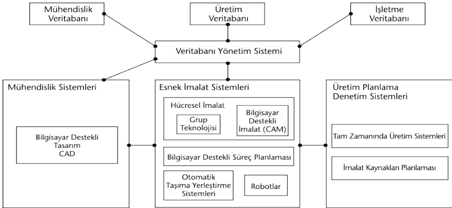
Şekil 2.5. Bir bilgisayar bütünleşik imalat sistemi genel yapısı (Eraslan, 2007)
