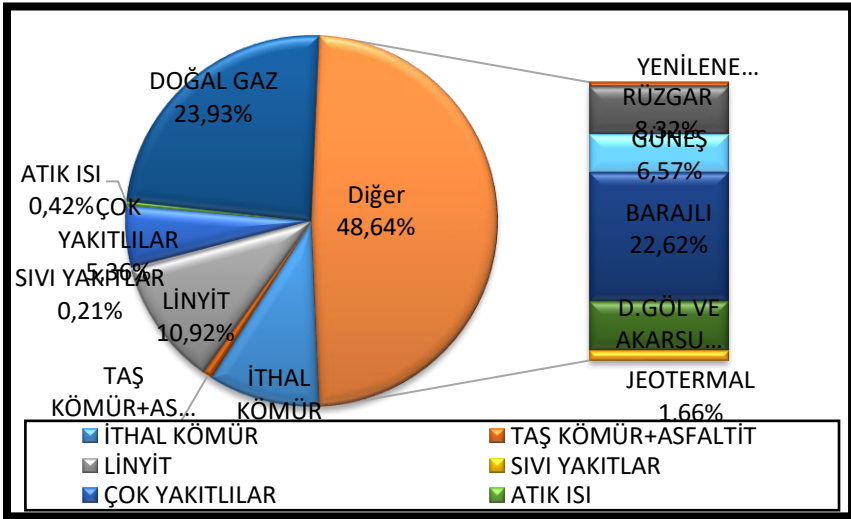
Şekil 3: 2019 Yılı Kurulu Gücünün Birincil Enerji Kaynaklarına Göre Dağılımı (MW)
