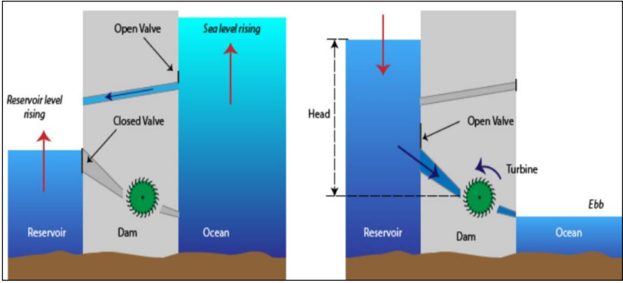
Şekil 4. Gelgit Aralığından Enerji Üretimi
