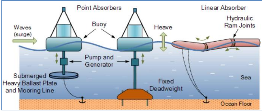
Şekil 7. Dalga Enerjisi Üretimi
