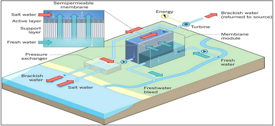
Şekil 6. Osmotik Enerji Üretimi. Kaynak: Logan ve Elimelech, 2012:314
