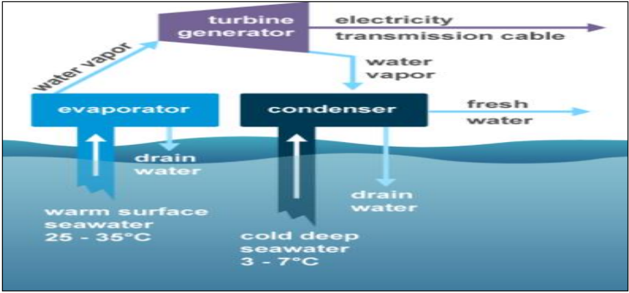
Şekil 3. OTEC Elektrik Enerjisi Üretim Sistemi
