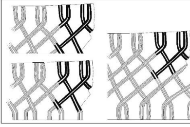
Çiz. 5: Zencirek İçin Üç Ayrı Örgü Önerisi
