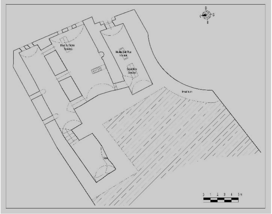
Çiz. 2: Ziyaretgâh Planı (Hatay Vakıflar Bölge Müdürlüğü Arşivinden İşlenerek)
