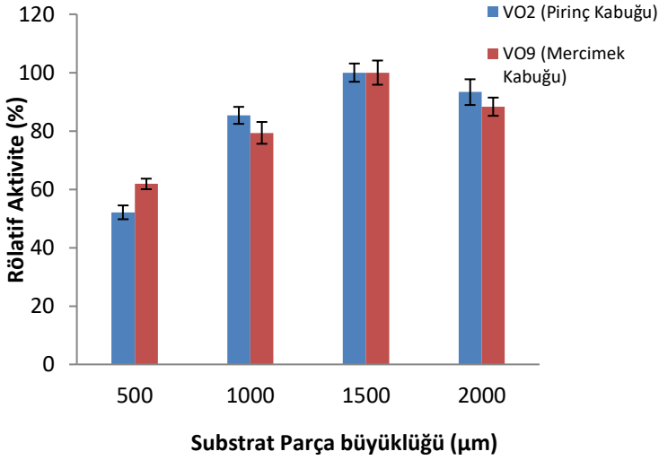
Şekil 4.13. \beta -galaktosidaz üretimi için uygun substrat büyüklüğünün tespit edilmesi
