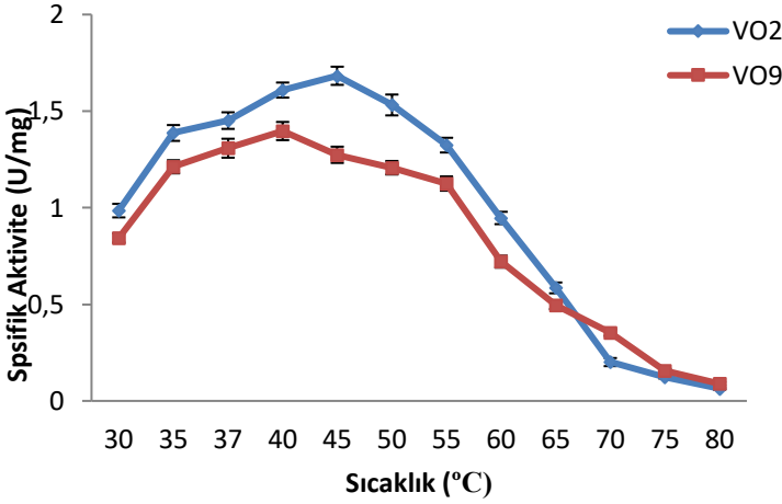
Şekil 4.16. Sıcaklığın 2 ve 9 nolu izolatlarda β-galaktosidaz üretimi üzerine etkisi
