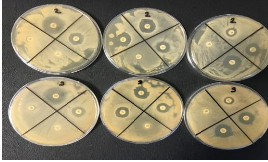
Şekil 4.5. Disk Diffüzyon Antibiyotik Testi
