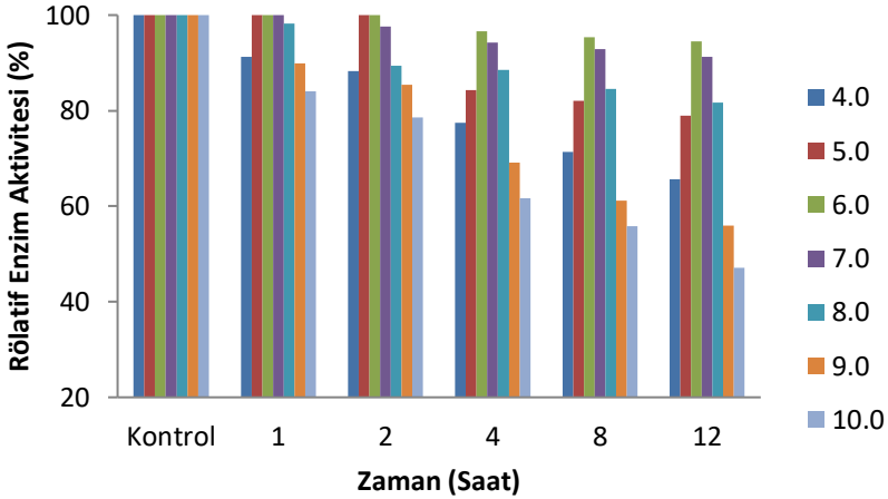
Şekil 4.25.VO2 izolatına ait β-galaktosidaz’ın zamana bağlı pH stabilitesi
