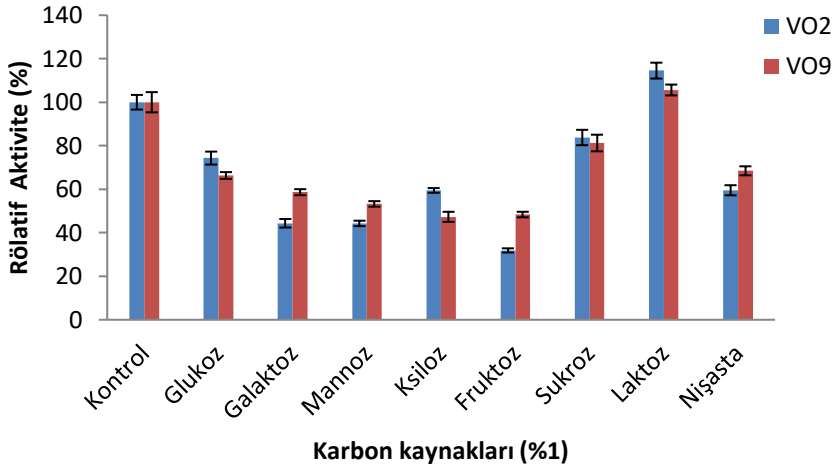
Şekil 4.19. Farklı karbon kaynaklarında β-galaktosidaz üretimi
