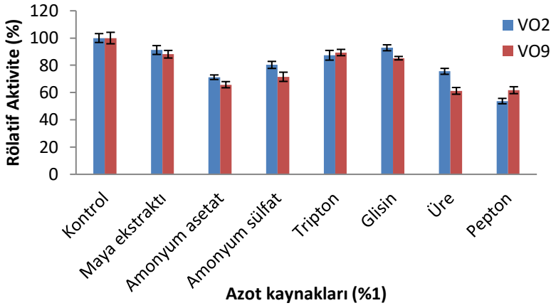
Şekil 4.20.Farklı azot kaynaklarında \beta -galaktosidaz üretimi
