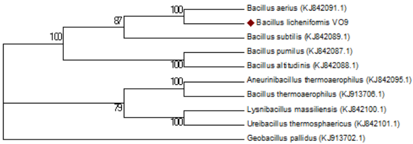
Şekil 4.6. İzolat VO2 ve VO9 'un yakın türler ile dendrogram gösterimi
