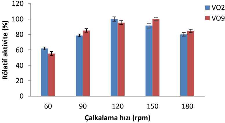
Şekil 4.15. \beta -galaktosidaz üretimi için uygun çalkalama hızı
