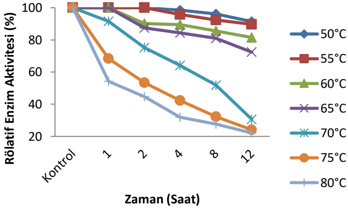
Şekil 4.23.VO2 izolatına ait \beta -galaktosidaz’ın zamana bağlı sıcaklık stabilitesi
