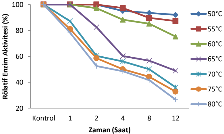
Şekil 4.24.VO9 izolatına ait \beta -galaktosidaz’ın zamana bağlı sıcaklık stabilitesi
