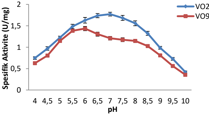
Şekil 4.17. pH'nın 2 ve 9 nolu izolatlarda β-galaktosidaz üretimi üzerine etkisi
