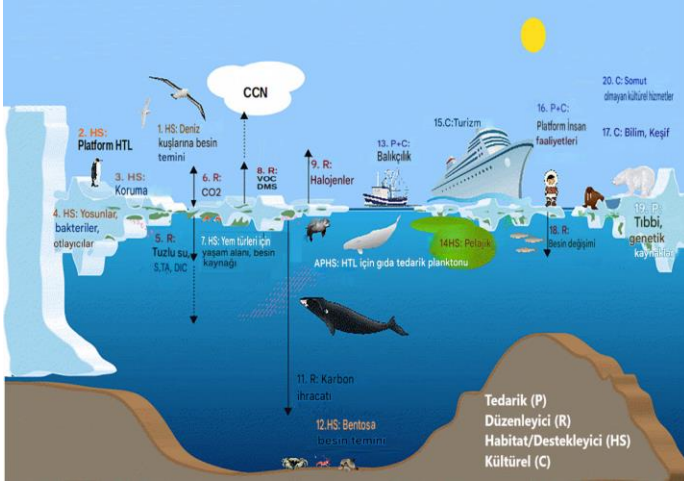
Şekil 13. Deniz buzı ekosistem hizmetlerinin temel örnekleri. Kutup deniz buzı ekosistemleri tarafından sağlanan tedarik (P), düzenleyici (R) habitat/destekleyici (H) ve kültürel (C) ekosistem hizmetlerine örnekler: (1) Daha yüksek trofik seviyedeki türlere ve deniz kuşlarına besin temini; (2) Daha yüksek trofik türlerin doğumu ve
