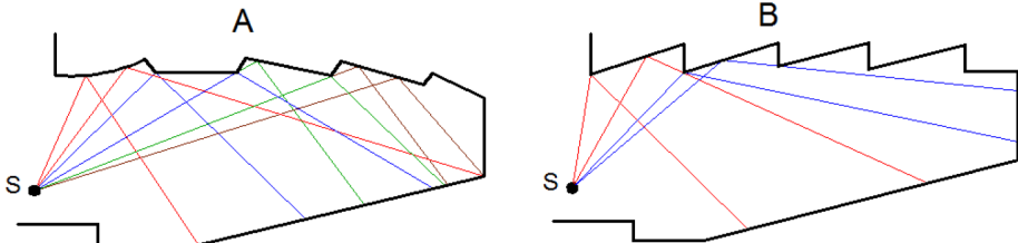
Şekil 3: Hacim akustiği bakımından iyi (A) ve kötü (B) tavan tasarımı örneği (Kanev, 2016)
